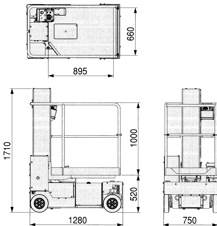
●車両寸法図(単位 m /m)
