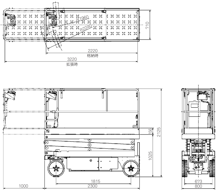
車両寸法図 (単位 m/m)
