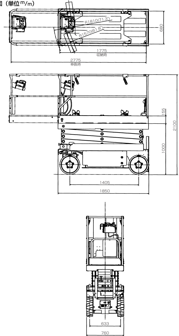
車両寸法図(単位m/m)
