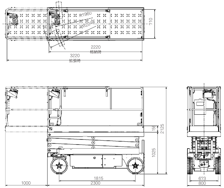
車両寸法図 (単位 m/m)
