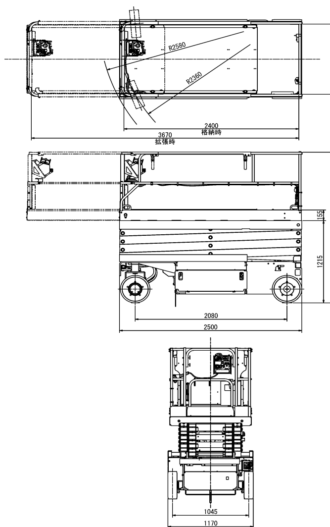
車両寸法図 (単位 m/m)
