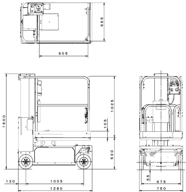
車両寸法図(単位m/m)
