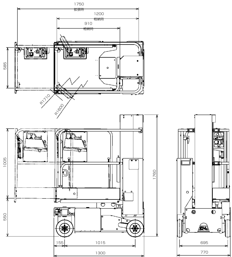
車両寸法図 (単位 m/m)
