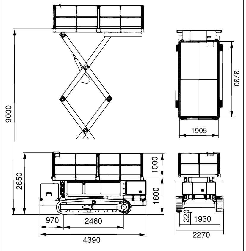
車両寸法図 (単位m/m)
