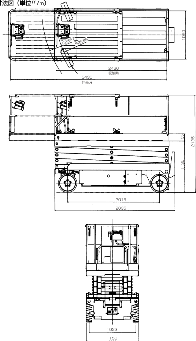
車両寸法図(単位m/m)
