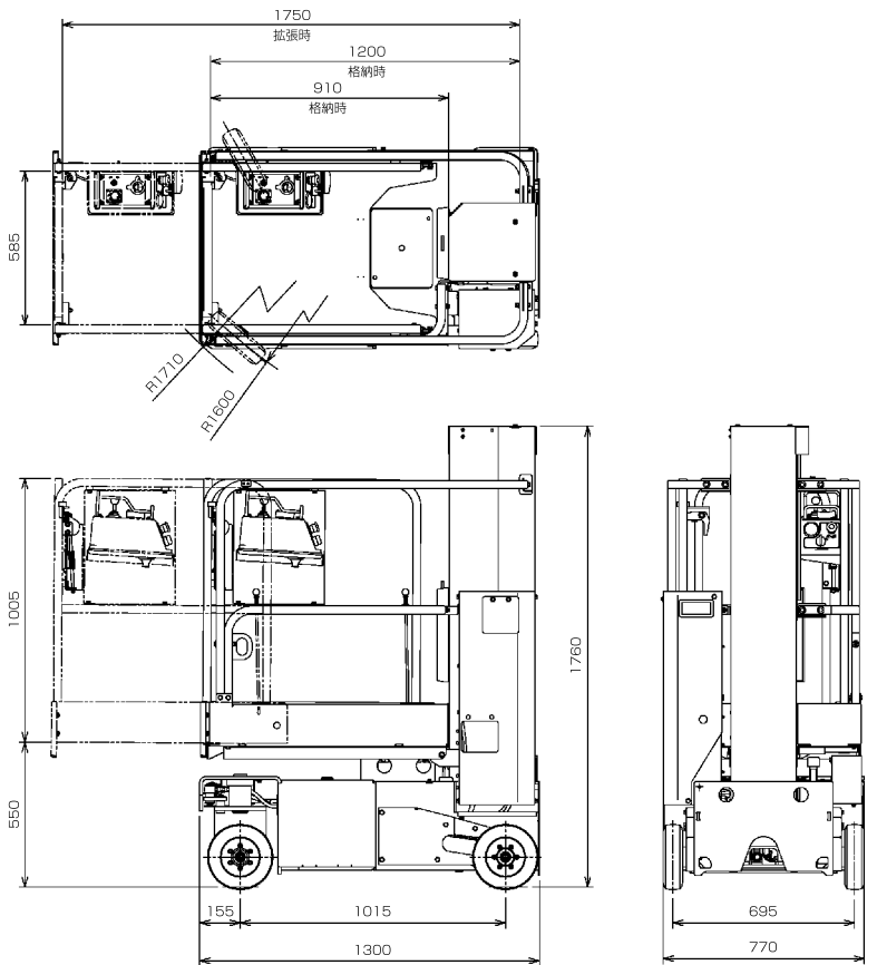
車両寸法図 (単位 m/m)
